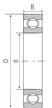
Bearings / Roulements
